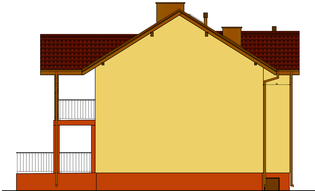
ELEWACJA POŁUDNIOWA SKALA 1:100
